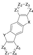
[화학식 4]
