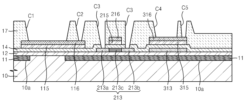
도면6
