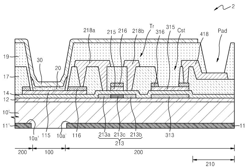
도면9
