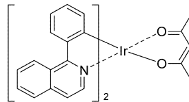
(piq) 2 Ir(acac)
