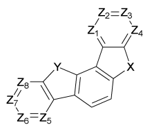
[화학식 4]
