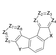
[화학식 5]
