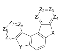
[화학식 5]
