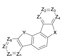
[화학식 4]
