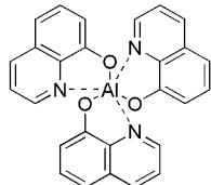
Alq
