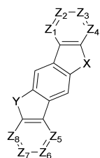
[화학식 4]
