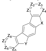
[화학식 3]
