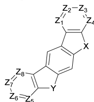
[화학식 3]
