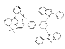
[화합물 218]
