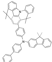
[화합물 101]
