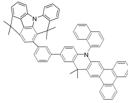
[화합물 119]
