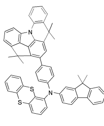
[화합물 8]
