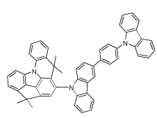
[화합물 240]
