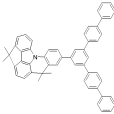
[화합물 193]
