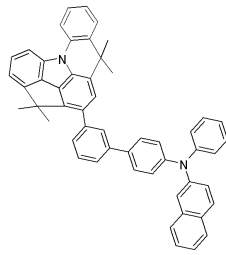
[화합물 35]
