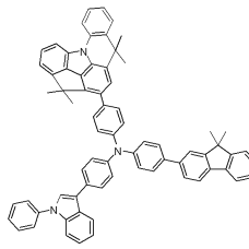
[화합물 66]
