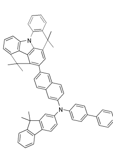
[화합물 48]
