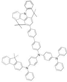
[화합물 61]
