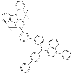
[화합물 37]
