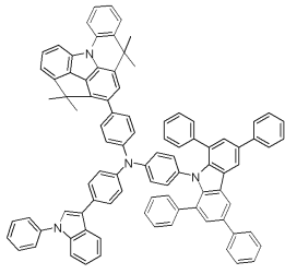
[화합물 70]
