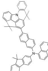
[화합물 102]
