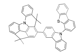
[화합물 221]
