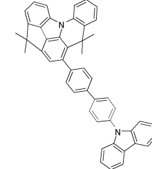
[화합물 140]
