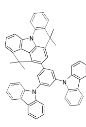
[화합물 21]
