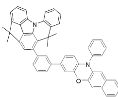
[화합물 115]
