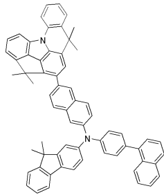
[화합물 47]
