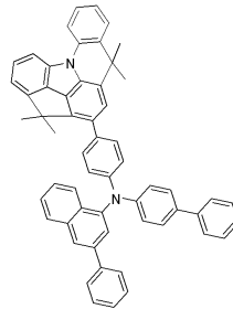
[화합물 30]
