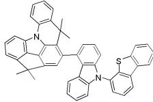
[화합물 178]
