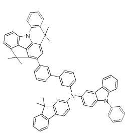
[화합물 46]
