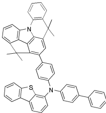
[화합물 28]
