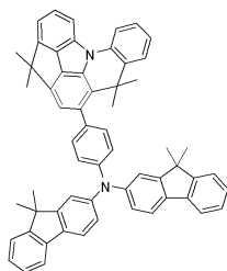
[화합물 100]
