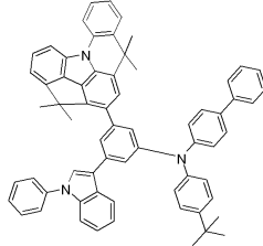
[화합물 89]
