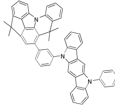
[화합물 134]
