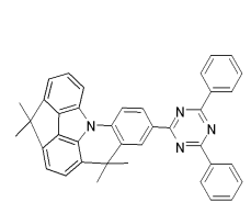
[화합물 186]
