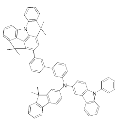
[화합물 56]
