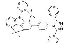
[화합물 223]
