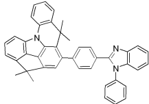
[화합물 201]
