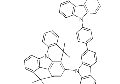
[화합물 241]
