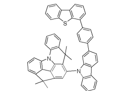
[화합물 238]
