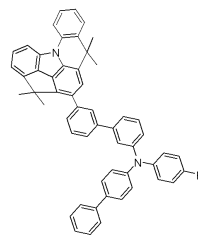
[화합물 39]
