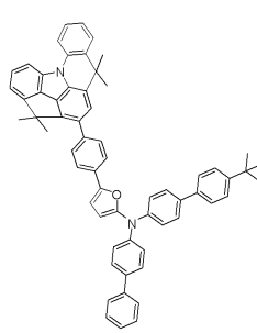
[화합물 57]
