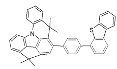
[화합물 206]
