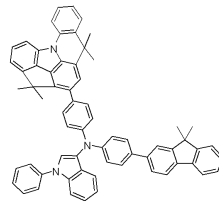
[화합물 75]
