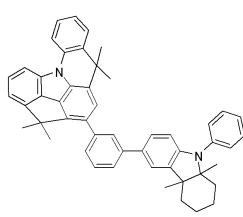
[화합물 109]
