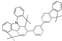
[화합물 198]
