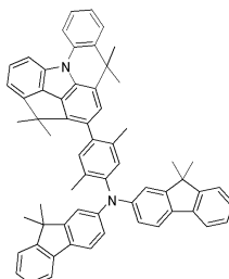
[화합물 11]
