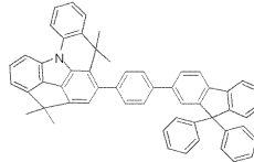
[화합물 197]
