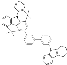
[화합물 111]
