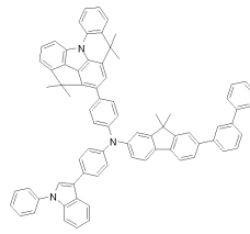
[화합물 63]
