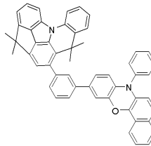
[화합물 116]
