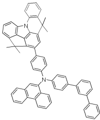
[화합물 85]
