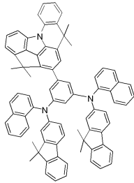
[화합물 95]
