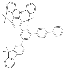
[화합물 144]
