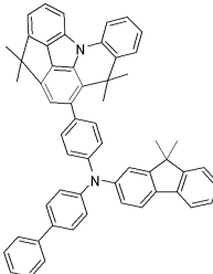
[화합물 101]
