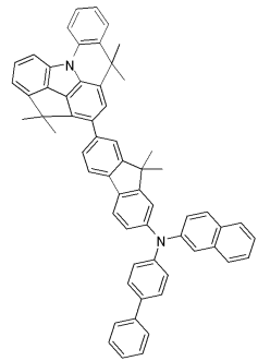
[화합물 47]
