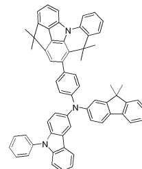
[화합물 102]
