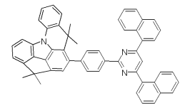
[화합물 152]
