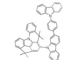
[화합물 241]
