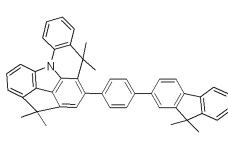
[화합물 196]
