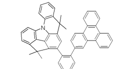
[화합물 155]
