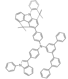
[화합물 65]
