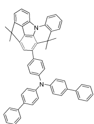
[화합물 100]
