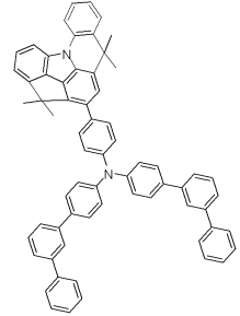
[화합물 86]
