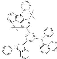
[화합물 99]
