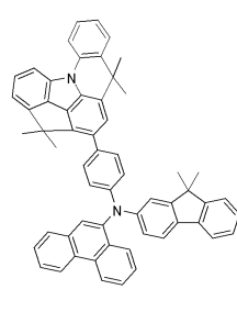
[화합물 21]
