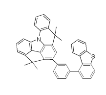
[화합물 182]
