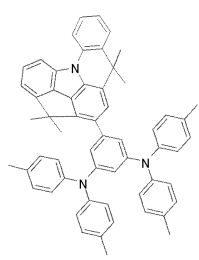
[화합물 19]
