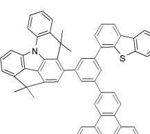
[화합물 188]
