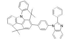
[화합물 200]
