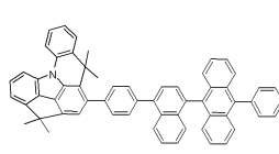
[화합물 203]
