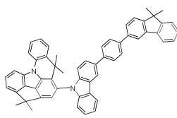
[화합물 230]
