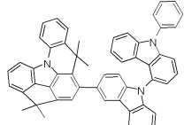
[화합물 222]
