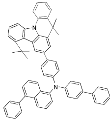
[화합물 29]
