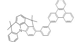
[화합물 215]
