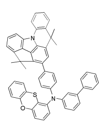
[화합물 10]
