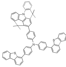
[화합물 62]
