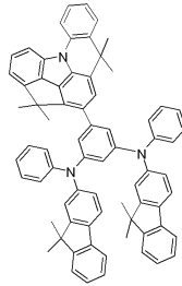
[화합물 96]
