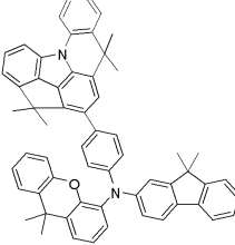
[화합물 10]
