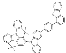
[화합물 237]
