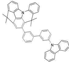
[화합물 139]
