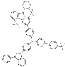
[화합물 64]
