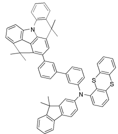
[화합물 37]
