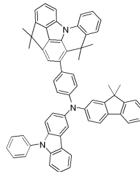
[화합물 102]
