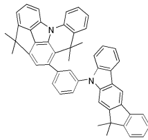
[화합물 138]
