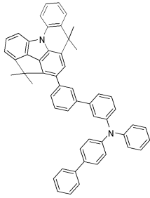
[화합물 43]
