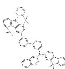
[화합물 39]
