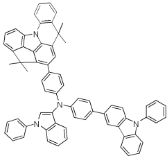
[화합물 76]
