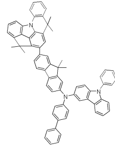
[화합물 48]
