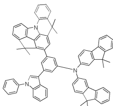
[화합물 88]
