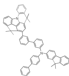
[화합물 38]
