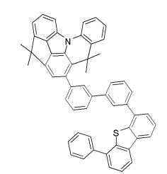
[화합물 140]
