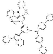
[화합물 90]
