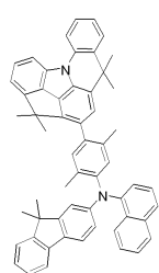
[화합물 101]
