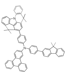
[화합물 76]
