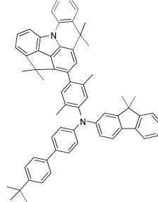
[화합물 18]
