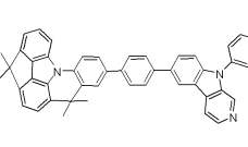
[화합물 205]
