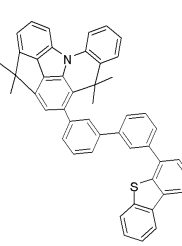
[화합물 139]
