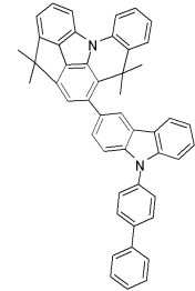
[화합물 138]
