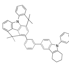
[화합물 110]
