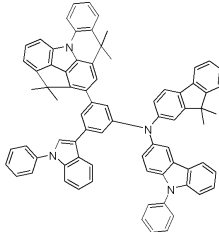
[화합물 89]
