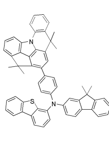
[화합물 20]
