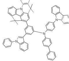
[화합물 90]
