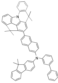
[화합물 16]
