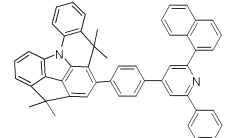
[화합물 154]
