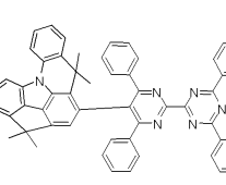
[화합물 242]
