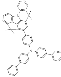
[화합물 84]
