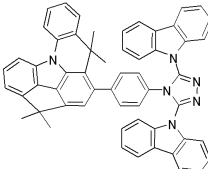
[화합물 219]
