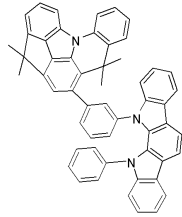
[화합물 133]
