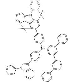
[화합물 65]
