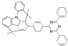
[화합물 147]
