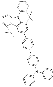
[화합물 34]
