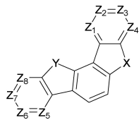
[화학식 4]
