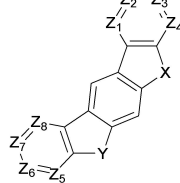
[화학식 3]
