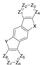
[화학식 4]
