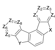
[화학식 5]
