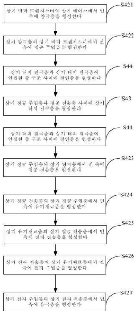
도면7
