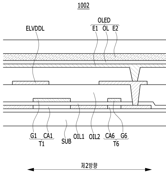
도면5
