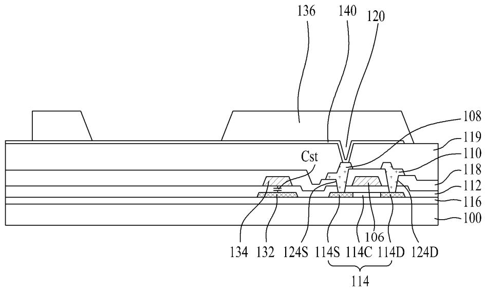
도면4i
