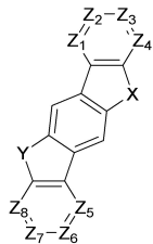
[화학식 4]
