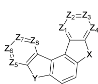
[화학식 5]
