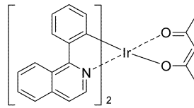
(piq) 2 Ir(acac)
