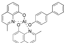
BALq
