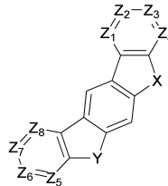
[화학식 3]
