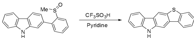
출발물질 S
