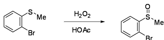
중간체 A
