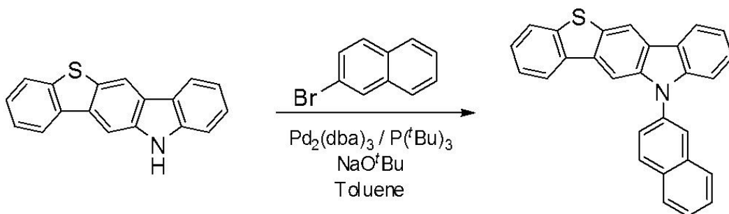
출발물질 S
