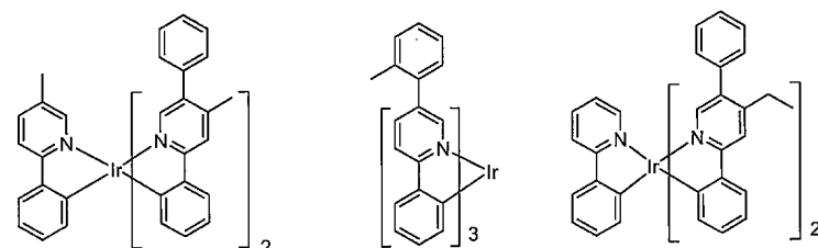
화합물 35
