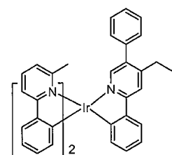
화합물 37
