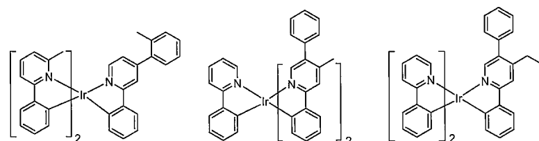
화합물 29
