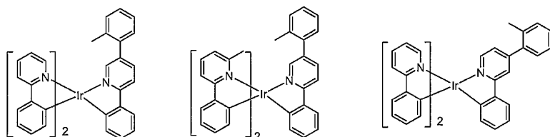
화합물 27
