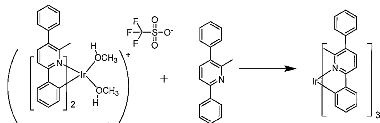
화합물 23
