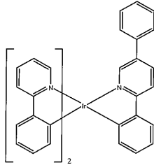
화합물 2
