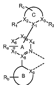
화합식 I.
