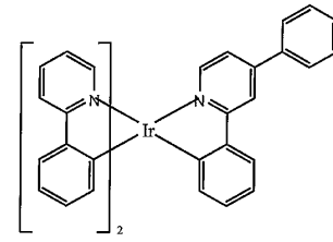
화합물 1
