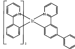
화합물 7
