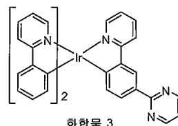
화합물 3
