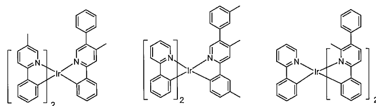
화합물 32
