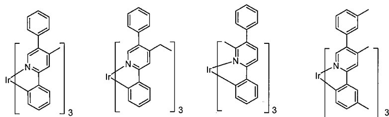
화합물 21
