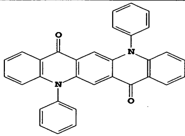
FD-45
