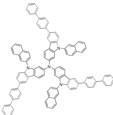
화합물 19
