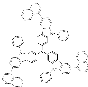
화합물 3
