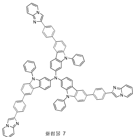
화합물 7
