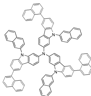
화합물 17
