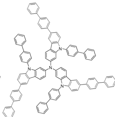
화합물 23
