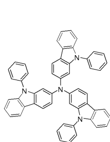
화합물 1
