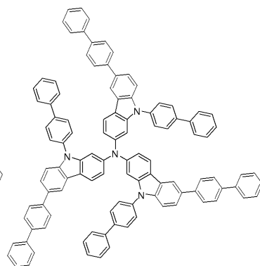
화합물 23
