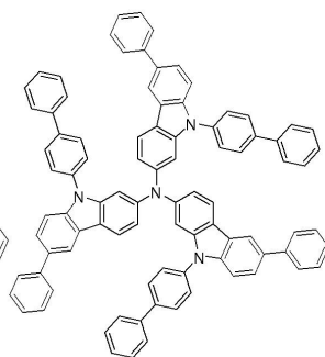
화합물 20
