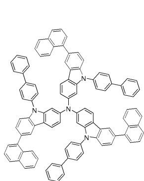
화합물 21
