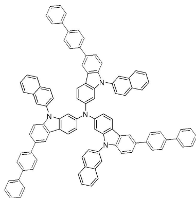
화합물 19
