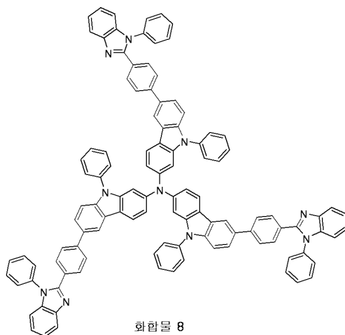
화합문 8
