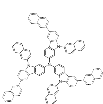
화합물 18
