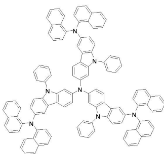
화합물 25
