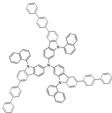
화합물 15
