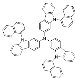
화한문 9
