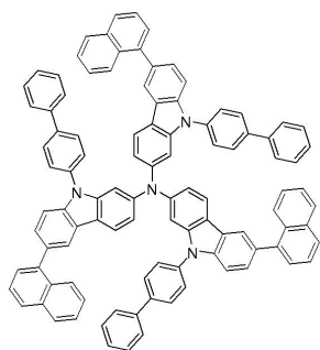
화합물 21
