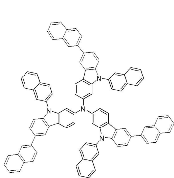
화합물 18
