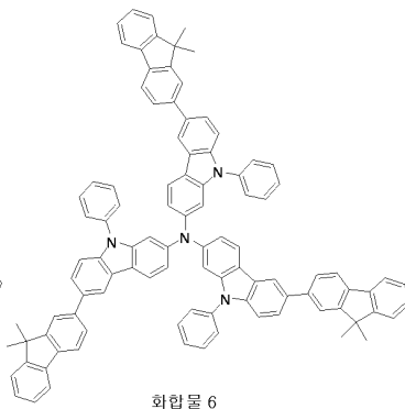
화합물 6
