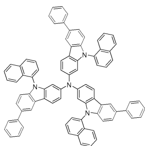
화합물 12
