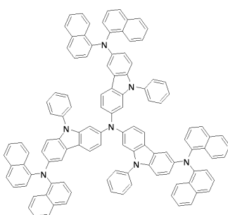
화합물 25
