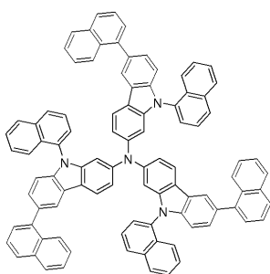
화합물 13
