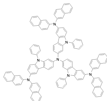
화합물 26
