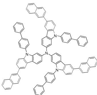
화합물 22
