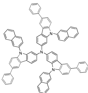
화합물 16
