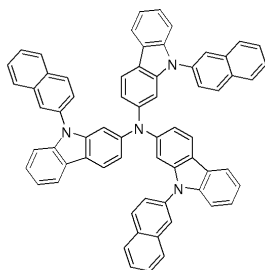
화합물 10
