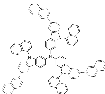
화합물 14
