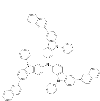
화합물 4
