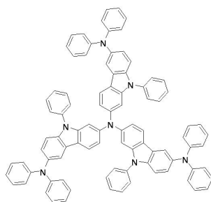
화합물 24
