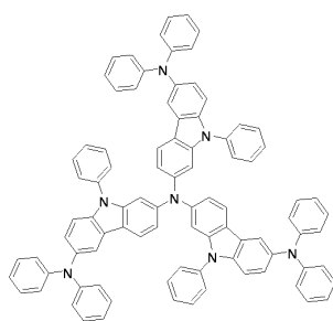
화합물 24
