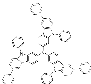
화합물 2
