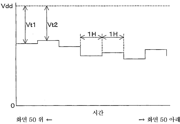
전류 Iw를 인가할 때의 소스 신호선 전위
