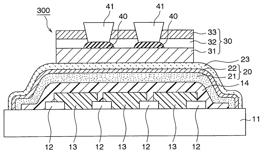
도면7
