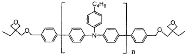
화합물 4
