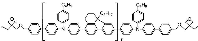
화합물 5
