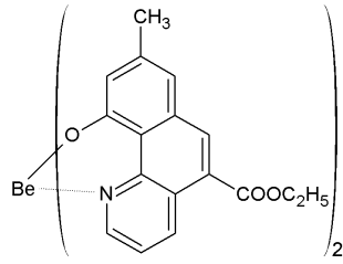
[화학식 2-19]
