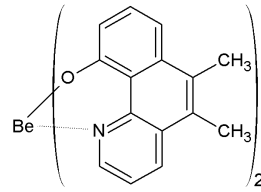
[화학식 2-6]
