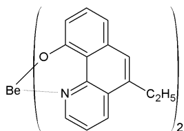
[화학식 2-7]
