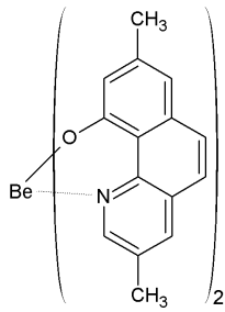
[화학식 2-18]
