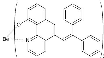
[화학식 2-17]
