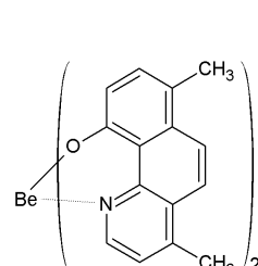
[화학식 2-12]
