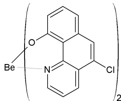
[화학식 2-13]
