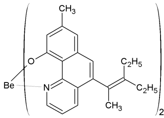
[화학식 2-20]
