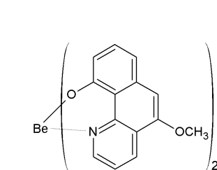
[화학식 2-11]
