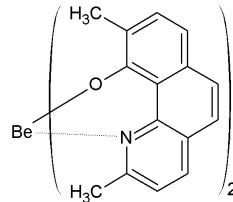
[화학식 2-12]
