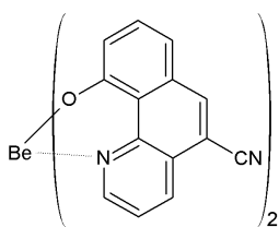
[화학식 2-14]
