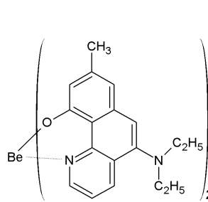
[화학식 2-17]
