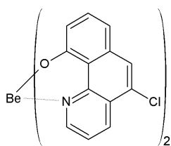
[화학식 2-13]
