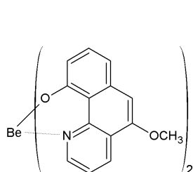
[화학식 2-11]
