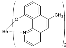
[화학식 2-5]
