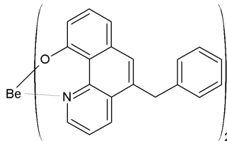
[화학식 2-15]
