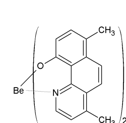
[화학식 2-12]
