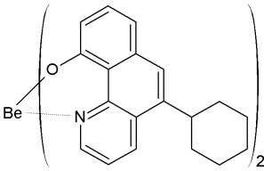
[화학식 2-8]
