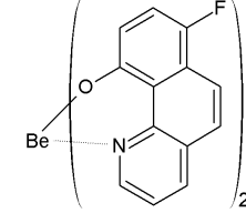
[화학식 2-9]
