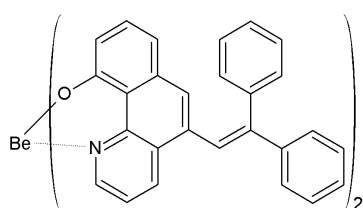
[화학식 2-17]
