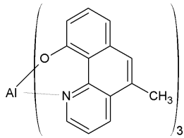
[화학식 2-20]
