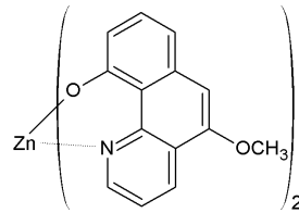
[화학식 2-21]
