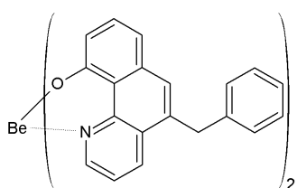
[화학식 2-15]
