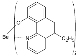
[화학식 2-7]
