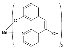
[화학식 2-4]
