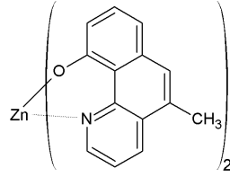
[화학식 2-21]
