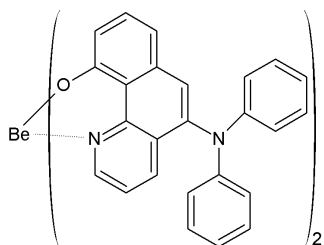
[화학식 2-10]
