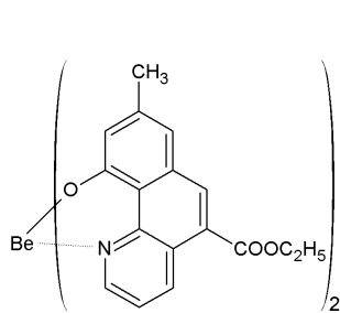
[화학식 2-19]
