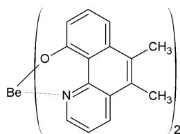
[화학식 2-6]
