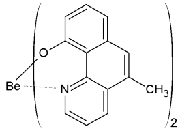
[화학식 2-4]
