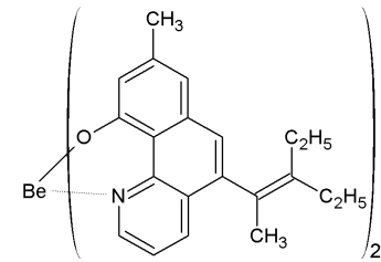
[화학식 2-20]
