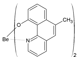
[화학식 2-5]
