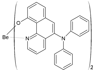
[화학식 2-10]
