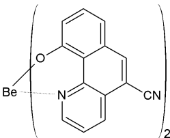
[화학식 2-14]
