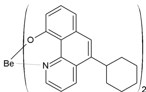
[화학식 2-8]
