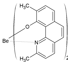
[화학식 2-12]
