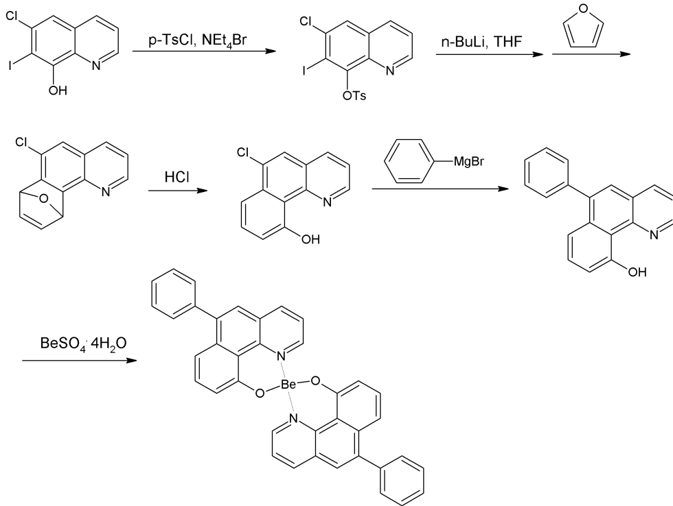
[화학식 3-5]
