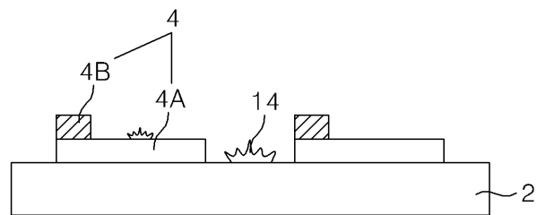
도면4a
