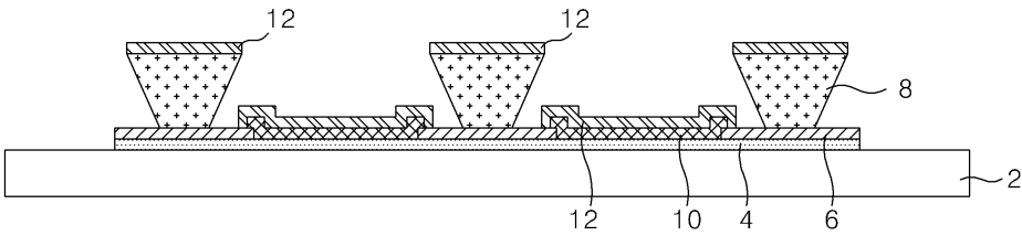
도면2
