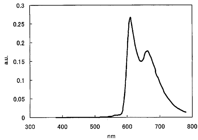
실시예 2의 EL 파형 ( 실시예 4,6도 동일파형 )
