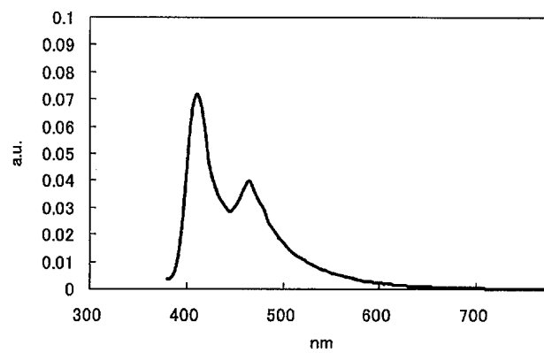
호스트1 발광파형 ( 비교예1 )
