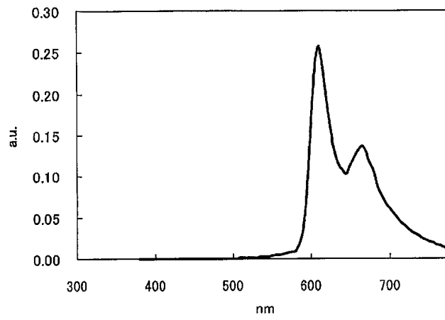
실시예 1의 EL 파형 ( 실시예 3,5도 동일파형 )
