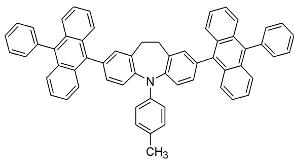
<화학식 11>
