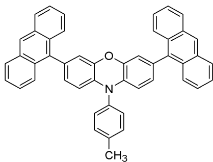
<화학식 10>
