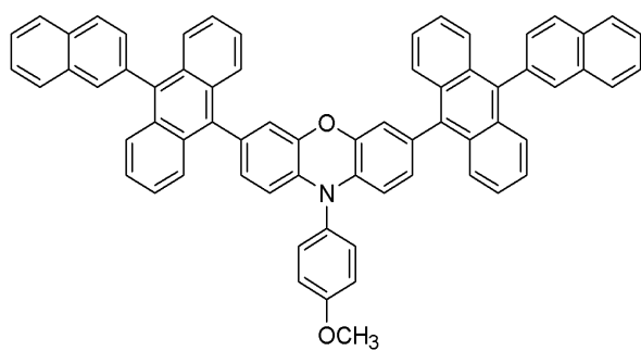
화학식 7
