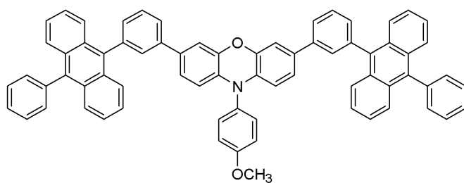
화학식 8
