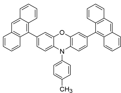
화학식 9
