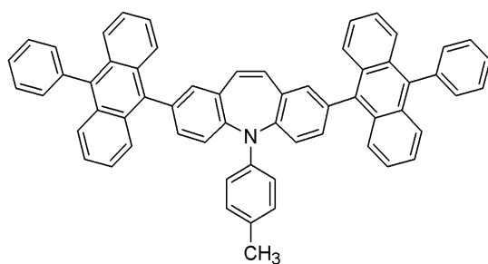
<화학식 11>
