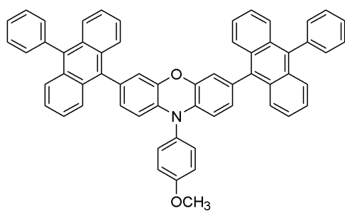
화학식 6
