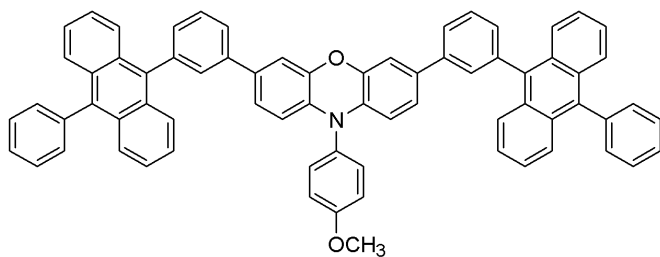
<화학식 9>
