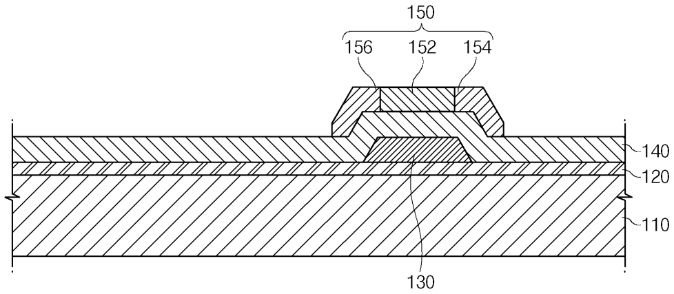
도면3e
