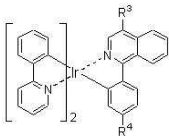
[화학식 4]
