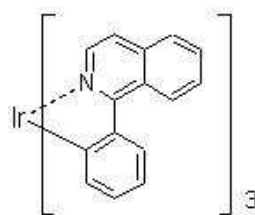
2-페닐이소퀴놀린 이리듐 착물
