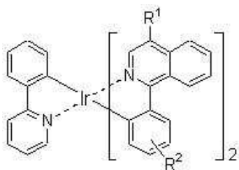
[화학식 2]
