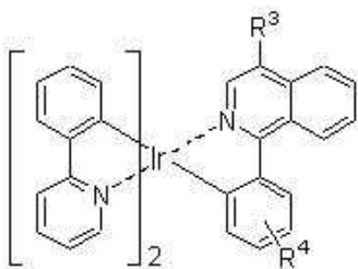
[화학식 2]
