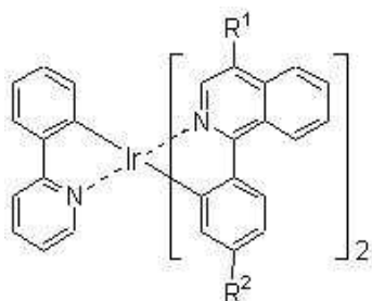
[화학식 4]
