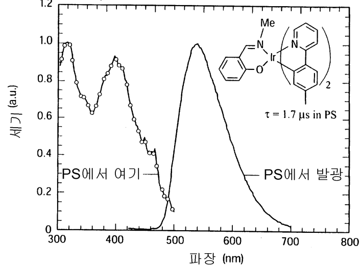
이리듐(III)비스(톨릴피리딘)살리실리덴 \text{tpylrdsd}
