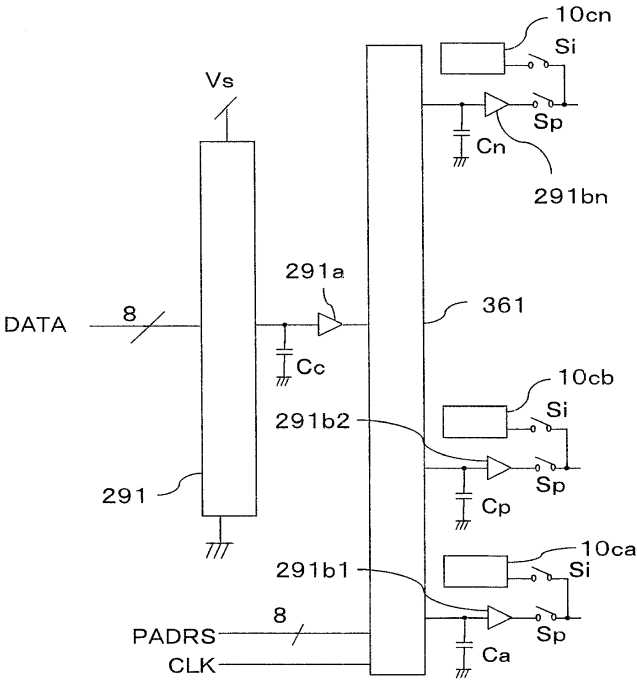
361 샘플 홀드
