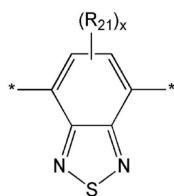
<화학식 13K>
