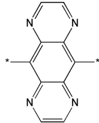
<화학식 13N>
