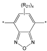
<화학식 13J>
