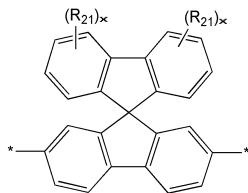
<화학식 13R>
