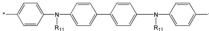
<화학식 13T>
