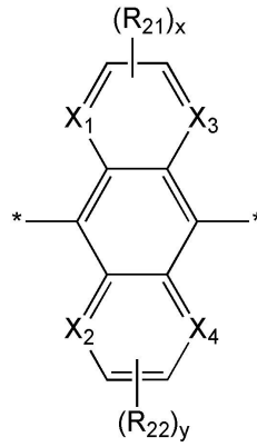
<화학식 12F>
