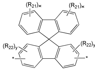
<화학식 12F>
