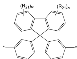
<화학식 13R>
