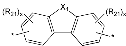
<화학식 12G>
