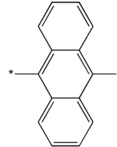
<화학식 13O>
