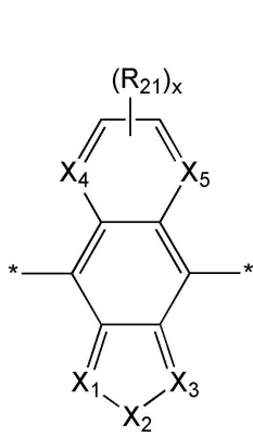
<화학식 12E>
