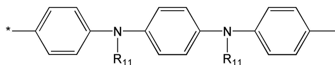
<화학식 13S>
