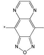
<화학식 13L>
