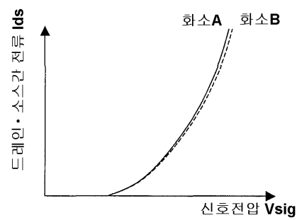
(c) 임계값 보정 : 있음, 이동도 보정 : 있음
