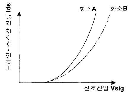
(b) 임계값 보정 : 있음, 이동도 보정 : 없음
