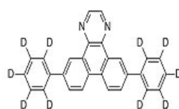
[화학식 10]
