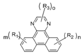
[화학식 1-a]
