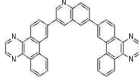
[화학식 84]
