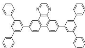
[화학식 9]
