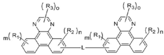
[화학식 1-b]
