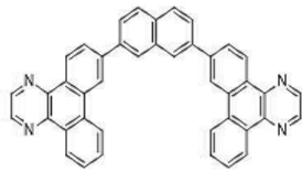
[화학식 83]
