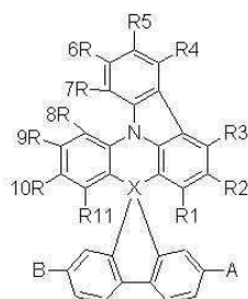
【화학식 2】
