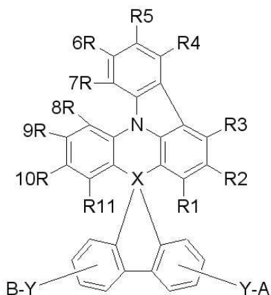
화학식 1
