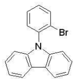
[화학식 a]
