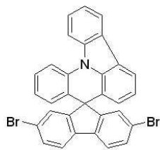
[화학식 b]
