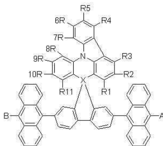
【화학식 5】
