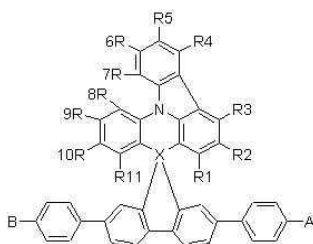
【화학식 3】
