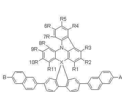
【화학식 4】
