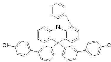
[화학식 c]
