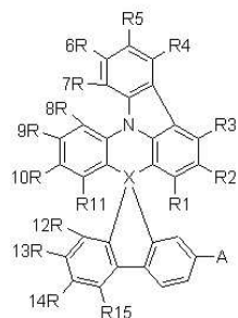
【화학식 2】
