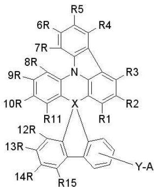
화학식 1
