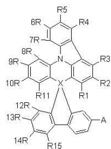
【화학식 2】
