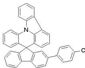
[화학식 c]
