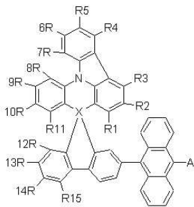
【화학식 5】
