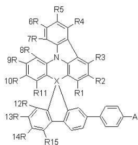
【화학식 3】
