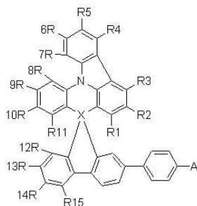
【화학식 3】
