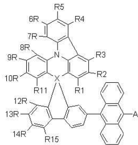
【화학식 5】
