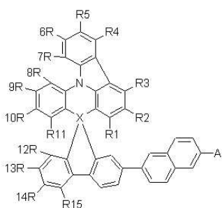
【화학식 4】
