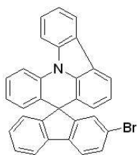
[화학식 b]
