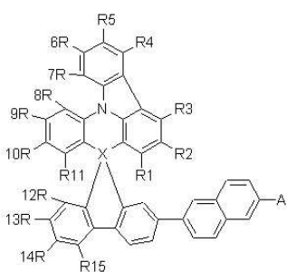
【화학식 4】
