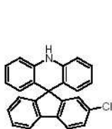
[화학식 a]
