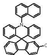
[화학식 b]
