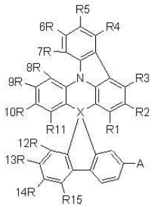
【화학식 2】
