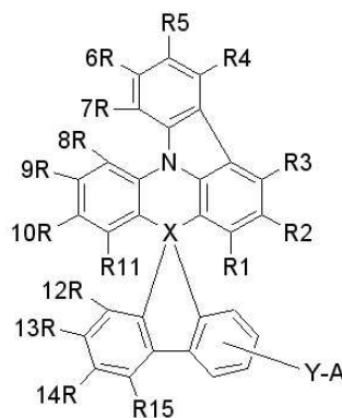
화학식 1
