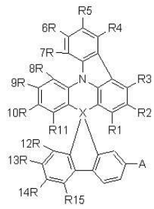
【화학식 2】
