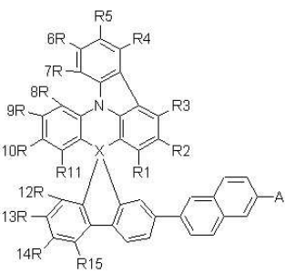
【화학식 4】
