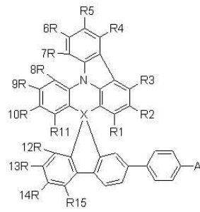
【화학식 3】
