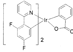
화학식 2
