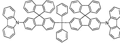
화학식 1e
