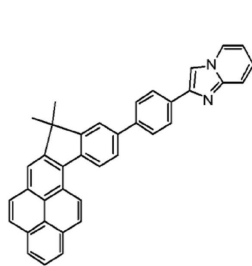
<화합물 14>
