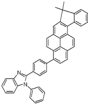
<화합물 7>
