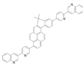
<화합물 33>
