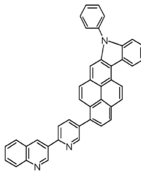
<화합물 18>
