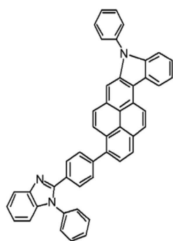
<화합물 19>
