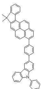
<화합물 41>
