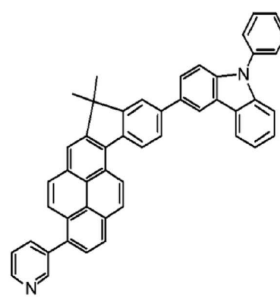
<화합물 24>
