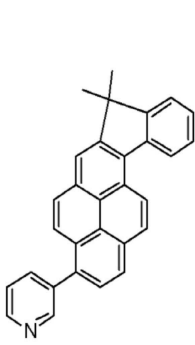
<화합물 4>
