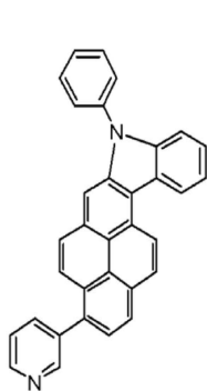
<화합물 16>
