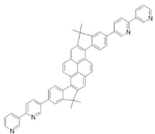
<화합물 32>
