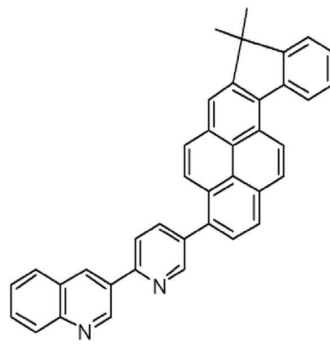
<화합물 6>
