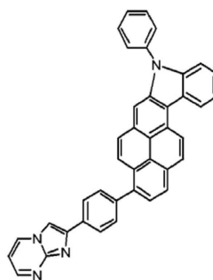
<화합물 21>
