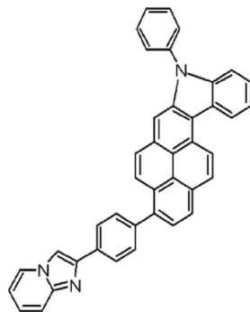
<화합물 20>
