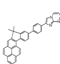
<화합물 15>
