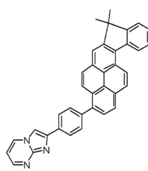
<화합물 9>
