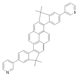
<화합물 31>
