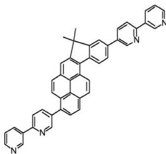
<화합물 23>
