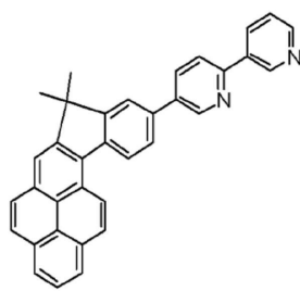
<화합물 11>
