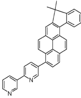
<화합물 5>
