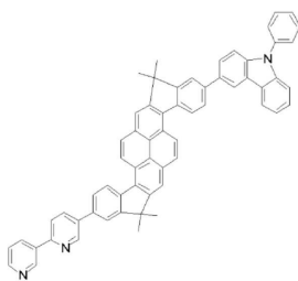
<화합물 35>
