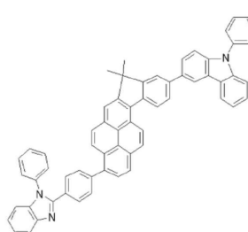
<화합물 27>
