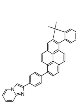
<화합물 8>
