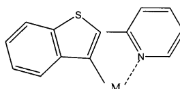
화학식 7
