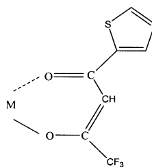
화학식 8
