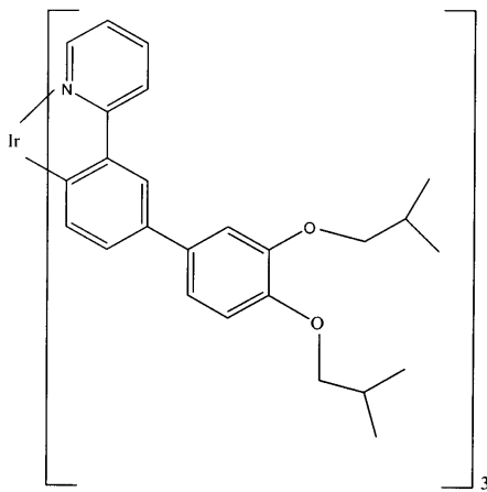
[화학식 15]
