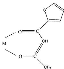
[화학식 9]
