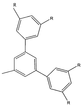
[화학식 13]
