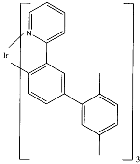
[화학식 15]
