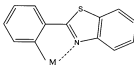
화학식 6
