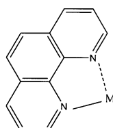
화학식 9
