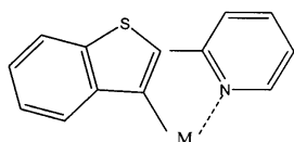
[화학식 8]
