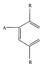
화학식 10
