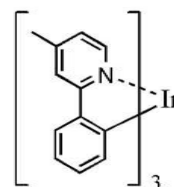
Ir(mppy) 3
