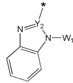
화학식 6Q
