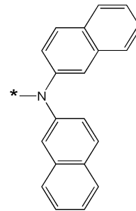
화학식 6Z
