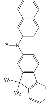
화학식 6V
