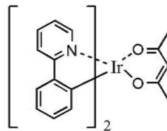
Ir(ppy) 2 (acac)
