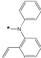
화학식 6T
