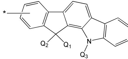
<화학식 3B-1>
