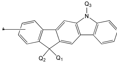
<화학식 3A-1>
