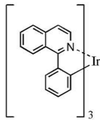
Ir(piq) 3
