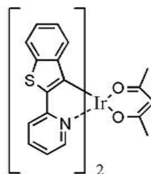
Btp 2 Ir(acac)
