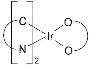
화학식 1
