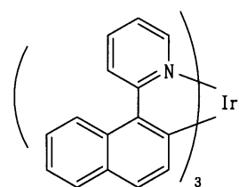
[화학식 27]
