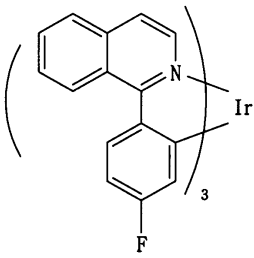
[화학식 30]
