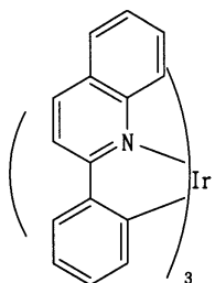
[화학식 29]
