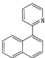
[화학식 5]
