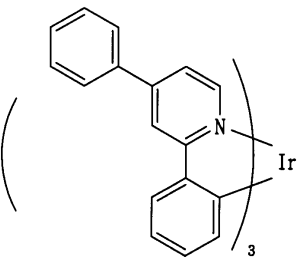
[화학식 31]
