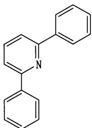
[화학식 14]
