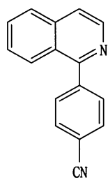
[화학식 12]
