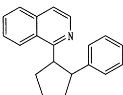
[화학식 14]
