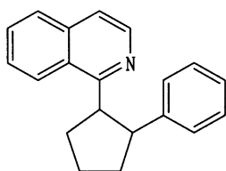
[화학식 15]
