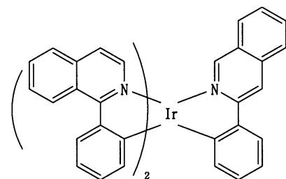
[화학식 21]
