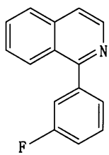
[화학식 13]
