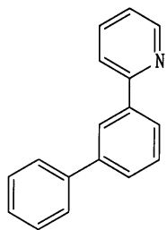
[화학식 4]
