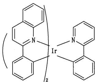
[화학식 17]
