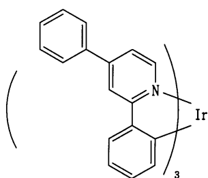
[화학식 31]
