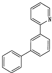
[화학식 4]
