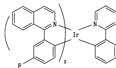
[화학식 20]
