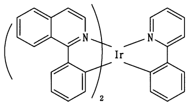
[화학식 18]
