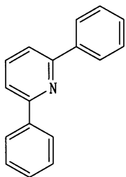
[화학식 14]
