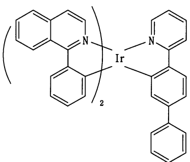
[화학식 22]
