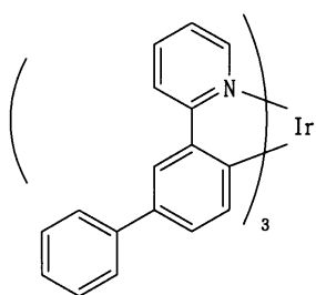
[화학식 26]
