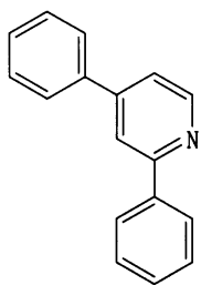
[화학식 9]
