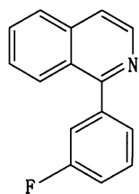
[화학식 12]
