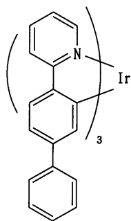
[화학식 25]
