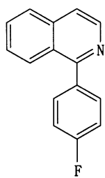
[화학식 8]
