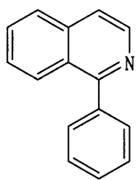
[화학식 6]
