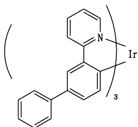
[화학식 26]
