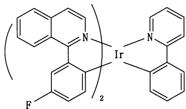
[화학식 20]
