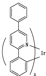
[화학식 14]
