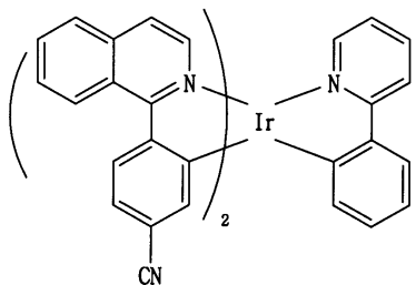
[화학식 19]
