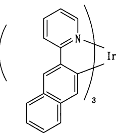
[화학식 31]
