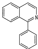
[화학식 6]
