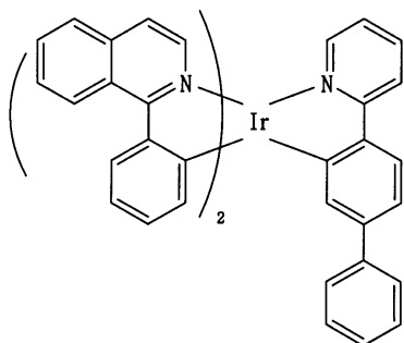
[화학식 22]
