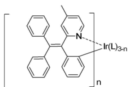
화학식 4f
