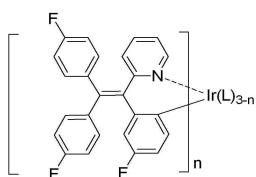
화학식 4g
