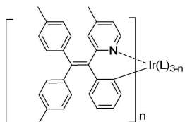
화학식 4e
