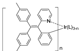
화학식 4b
