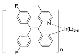
화학식 4d
