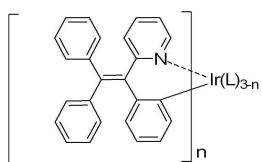
화학식 4c
