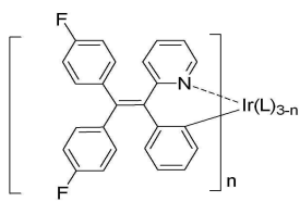
화학식 4a
