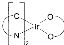
화학식 1
