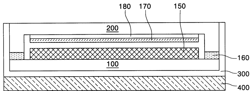
도면1b
