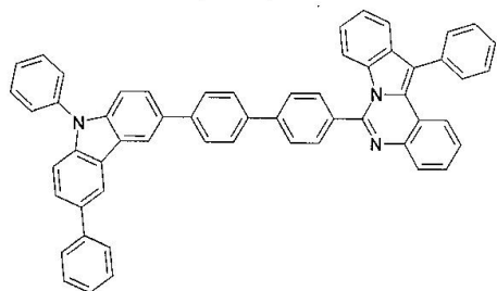
구조식 25
