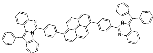
구조식 47
