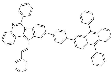
구조식 37
