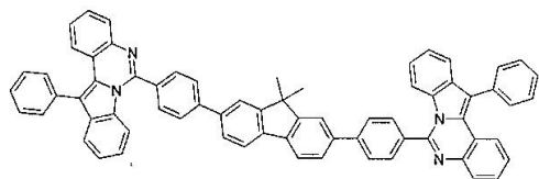
구조식 21
