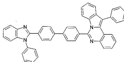
구조식 16
