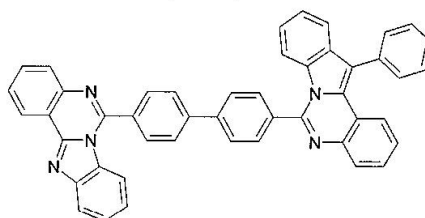
구조식 18
