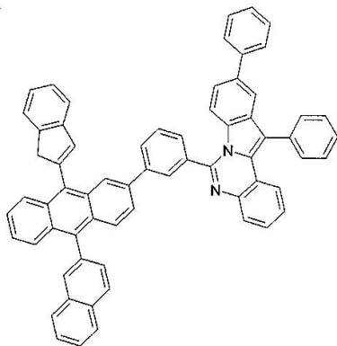
구조식 33
