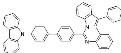
구조식 24
