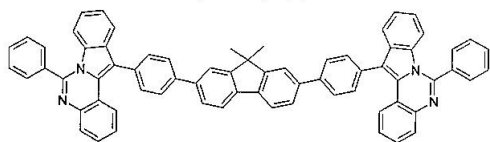
구조식 67
