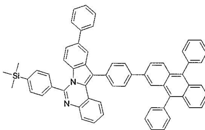
구조식 28
