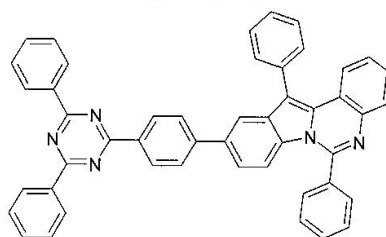
구조식 70
