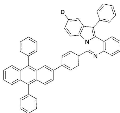
구조식 7
