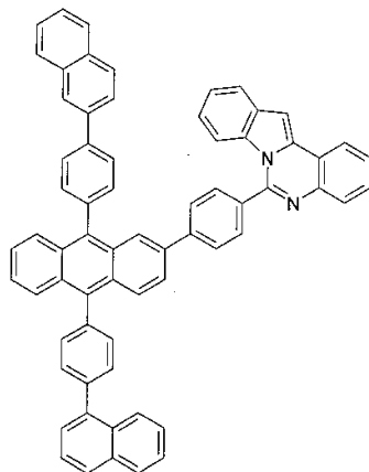
구조식 3
