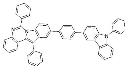
구조식 54
