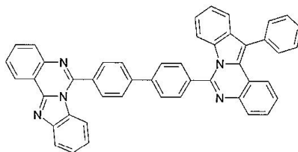
구조식 18
