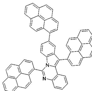
구조식 48
