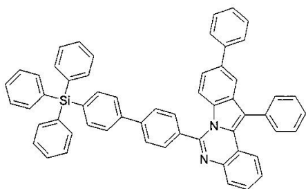
구조식 9
