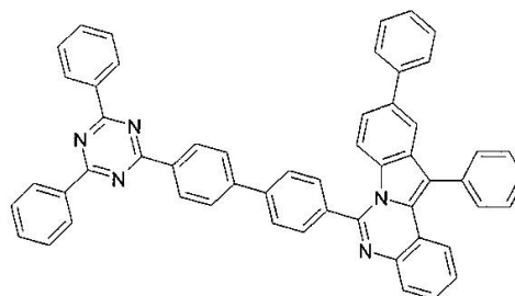
구조식 10
