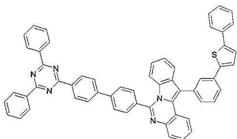
구조식 11
