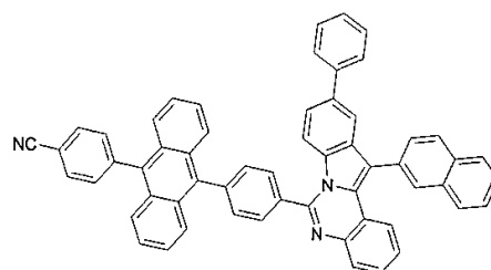
구조식 52
