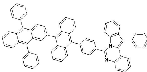
구조식 12
