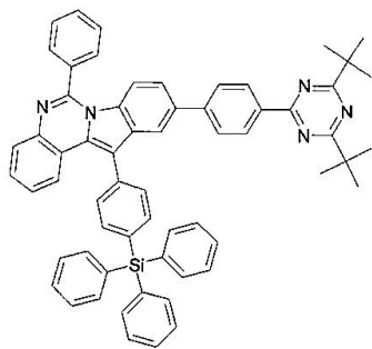
구조식 57
