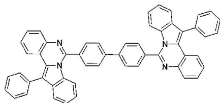
구조식 15
