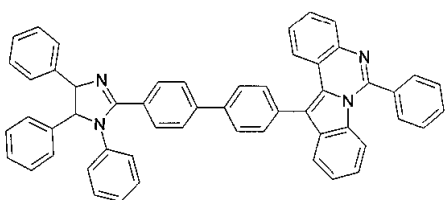
구조식 45
