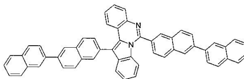
구조식 44
