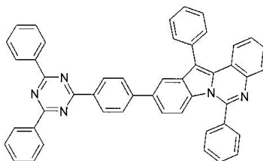
구조식 70
