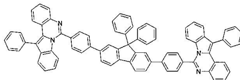
구조식 22
