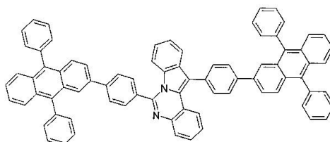
구조식 58
