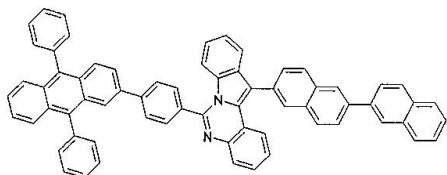
구조식 59
