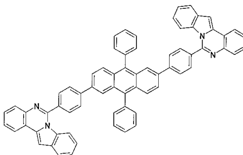
구조식 4
