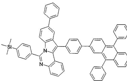
구조식 28
