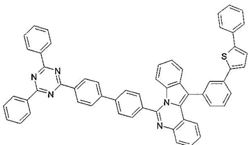
구조식 11
