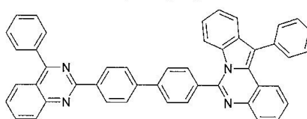
구조식 20
