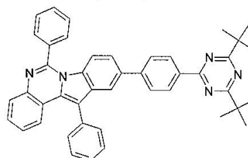
구조식 56
