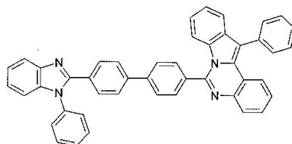
구조식 16
