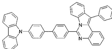
구조식 24
