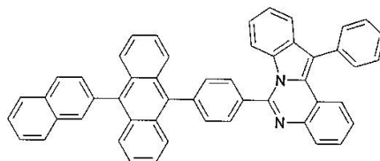
구조식 14
