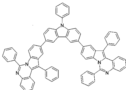
구조식 55
