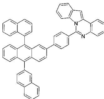
구조식 2
