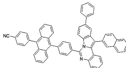
구조식 52
