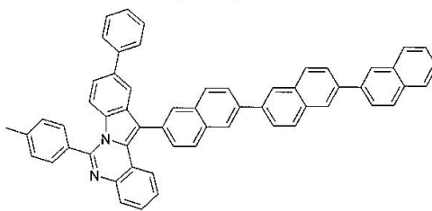
구조식 34
