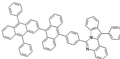
구조식 12
