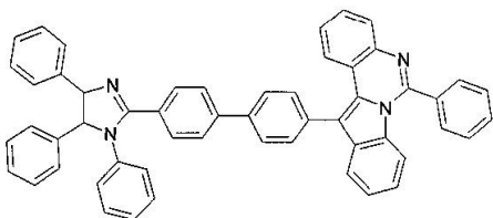
구조식 45
