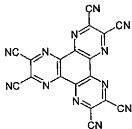
[헥사니트릴 헥사아자트리페닐렌]
