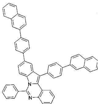
구조식 65
