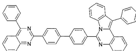
구조식 20
