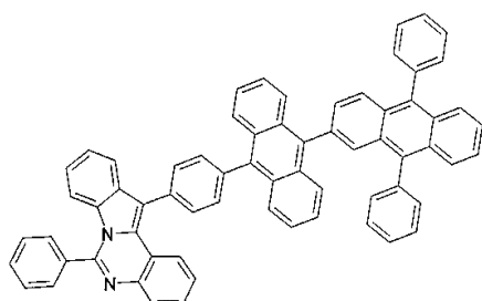
구조식 63
