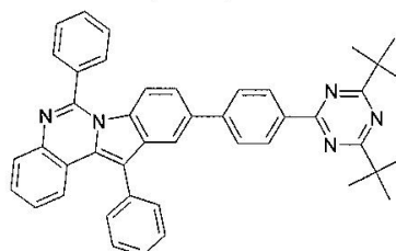
구조식 56
