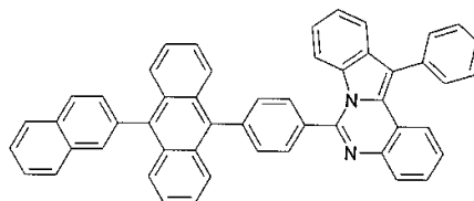
구조식 14
