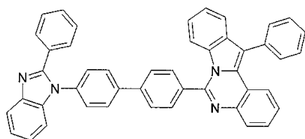
구조식 17
