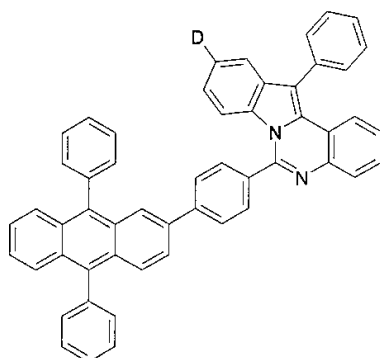
구조식 7
