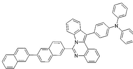
구조식 26
