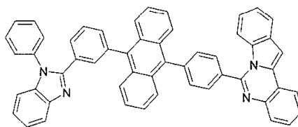
구조식 46
