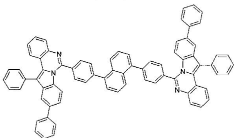
구조식 27
