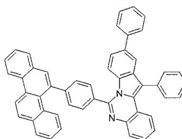
구조식 32
