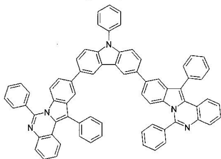
구조식 55
