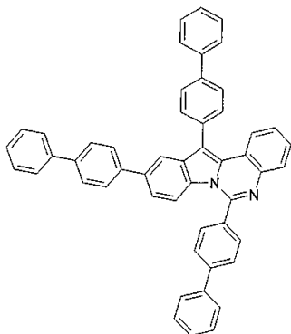
구조식 41
