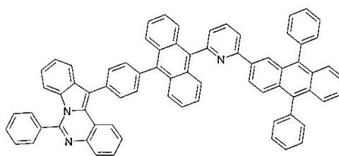
구조식 64
