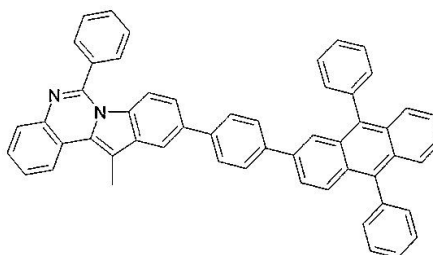
구조식 38
