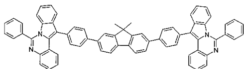
구조식 67
