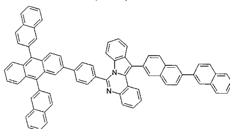
구조식 60
