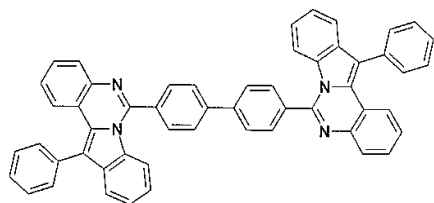
구조식 15
