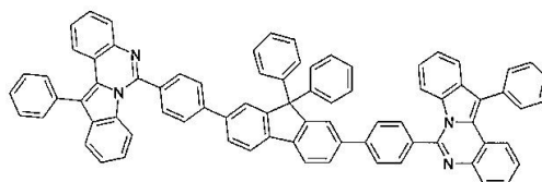
구조식 22
