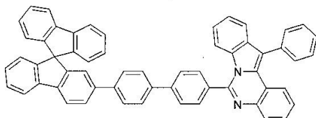
구조식 23
