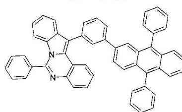
구조식 62
