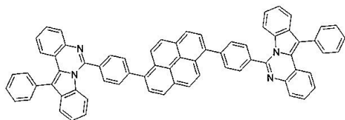
구조식 47
