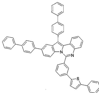
구조식 42
