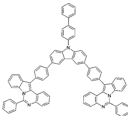
구조식 68
