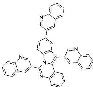
구조식 49
