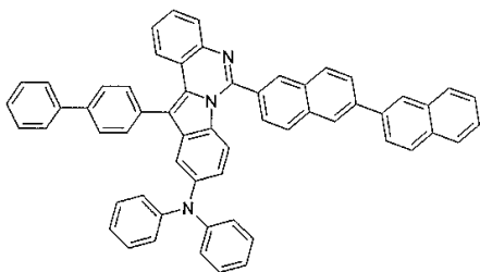
구조식 43
