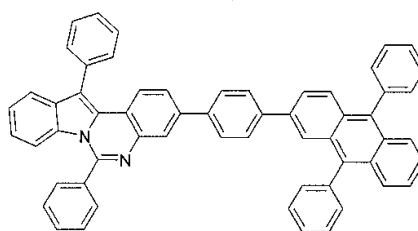
구조식 72
