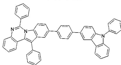
구조식 54
