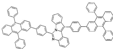
구조식 58
