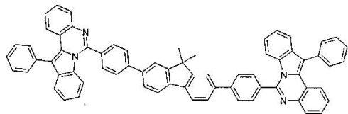
구조식 21
