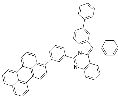
구조식 31
