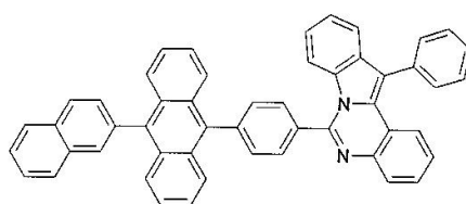
구조식 14
