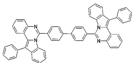
구조식 15
