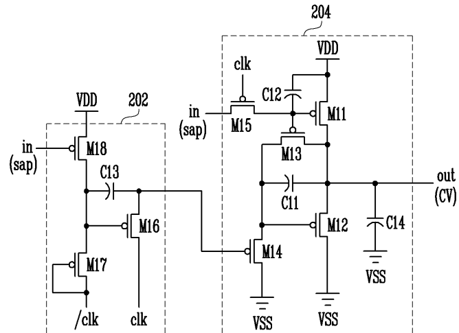
도면11
