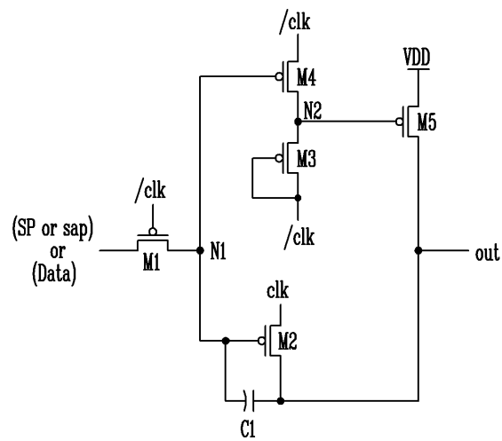
도면12
