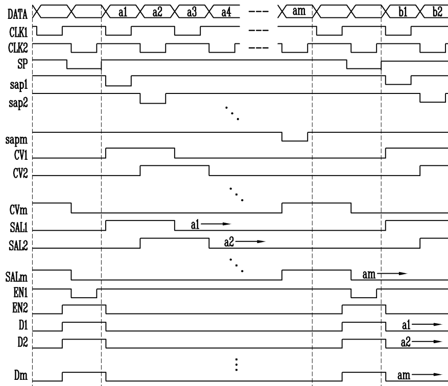
도면6
