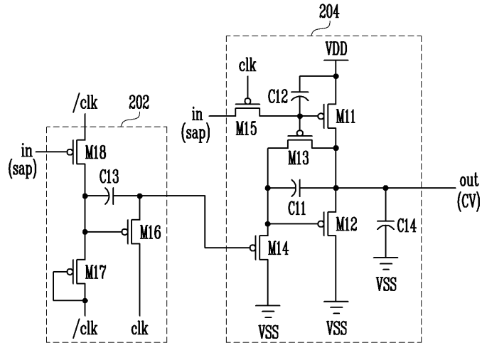
도면14
