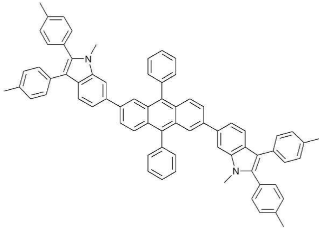
<화학식 8>
