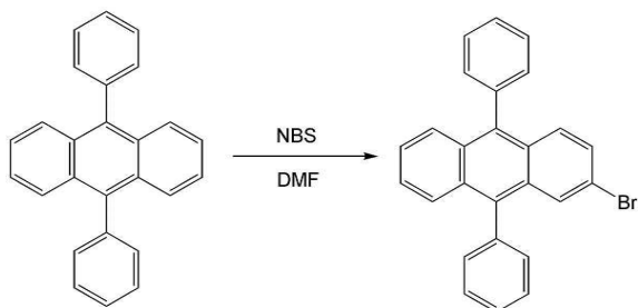
중간체 C
