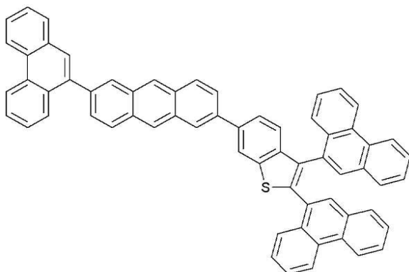
<화학식 25>
