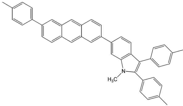
<화학식 12>
