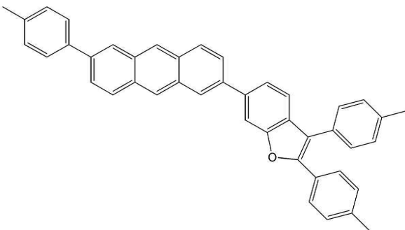
<화학식 10>
