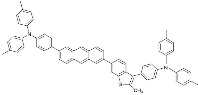
<화학식 23>
