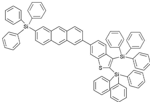
<화학식 25>
