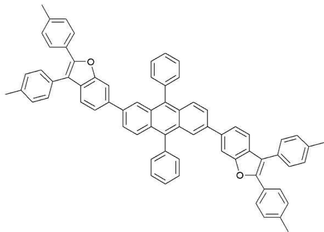
<화학식 6>
