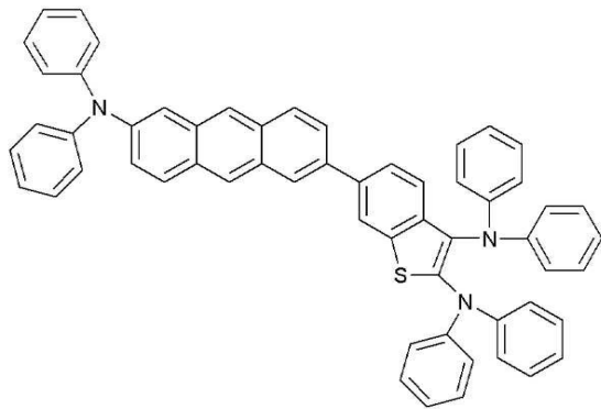
<화학식 20>
