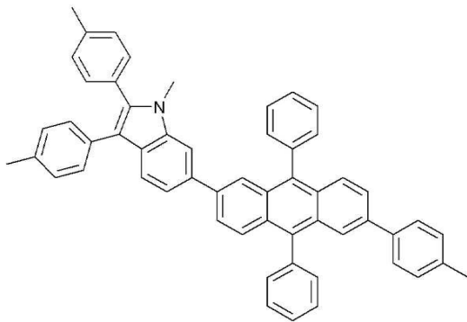
<화학식 8>
