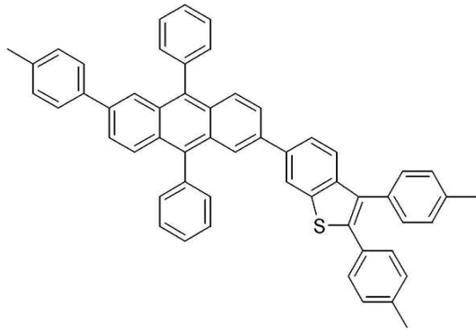
<화학식 5>
