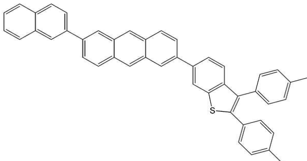
<화학식 14>
