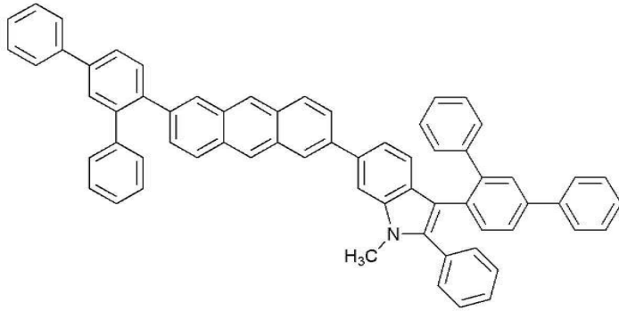
<화학식 19>
