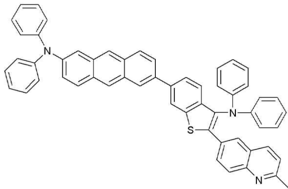
<화학식 21>
