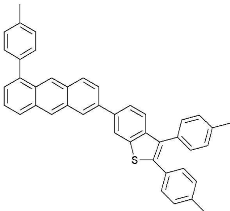
<화학식 17>
