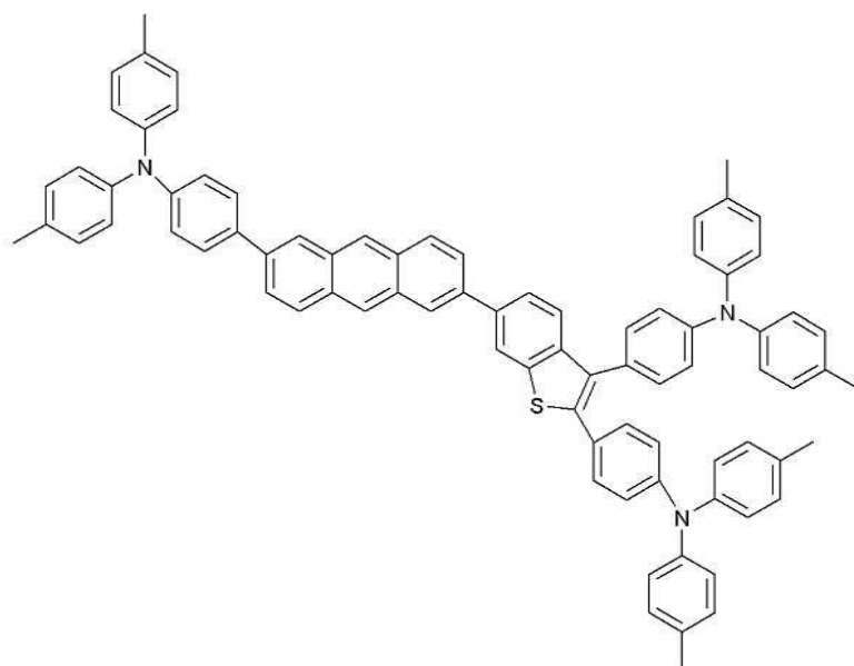
<화학식 14>
