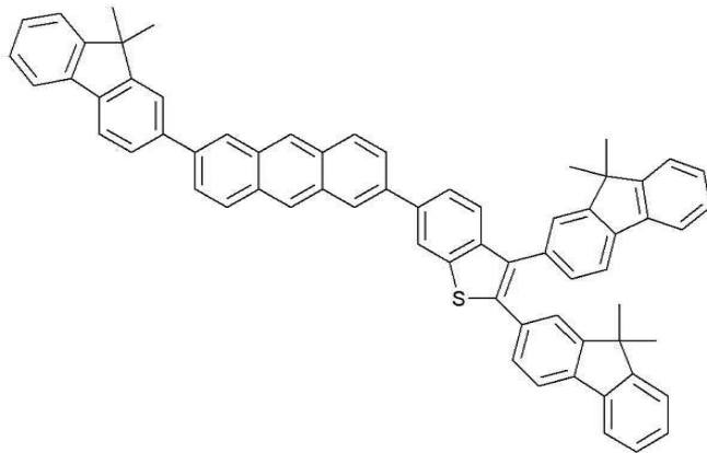
<화학식 24>
