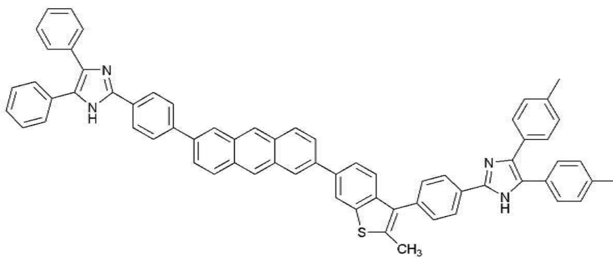
<화학식 21>
