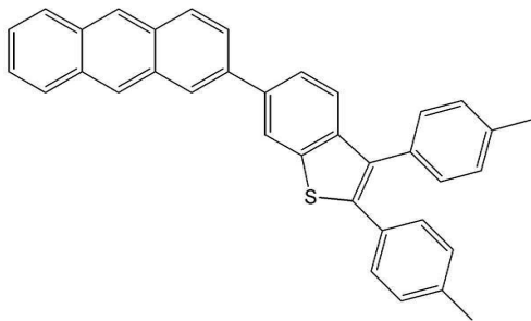
<화학식 13>
