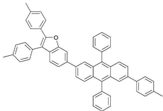
<화학식 6>
