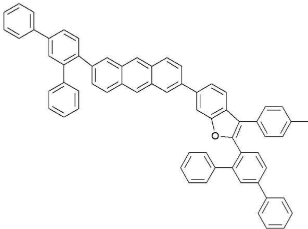
<화학식 17>
