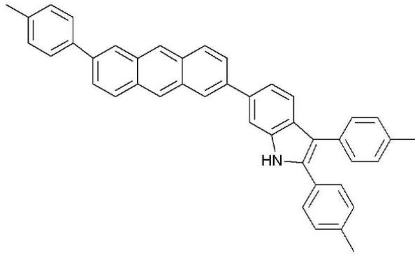
<화학식 16>
