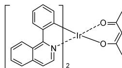
(piq) 2 Ir(acac)
