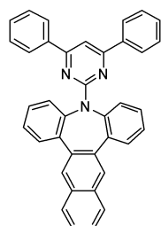
화합물 41
