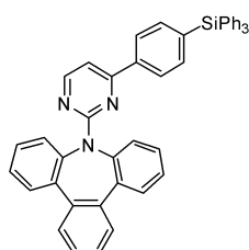
화합물 34
