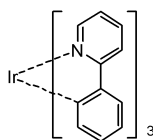
Ir(ppy) 3
