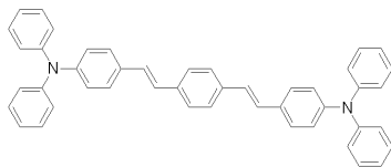
화합물 D
