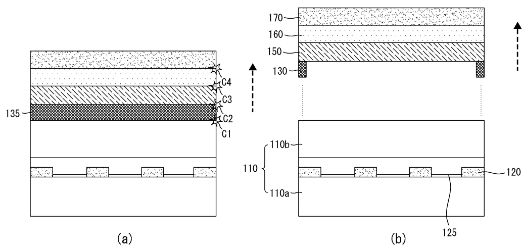
도면8
