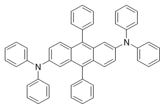
화합물 G
