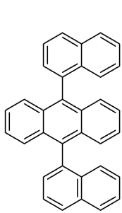
화합물 K
