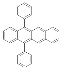
화합물 F
