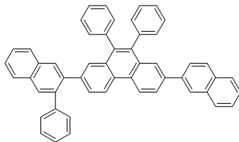
화합물 218
