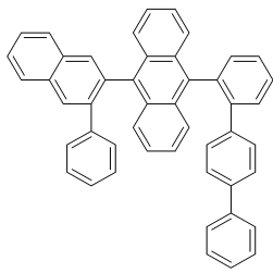
화합물 705
