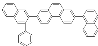
화합물 2
