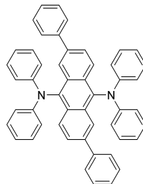
화합물 A
