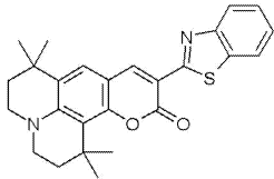
C545T
