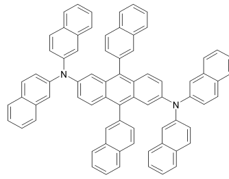
화합물 E
