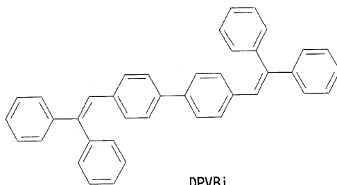
DPVBi
