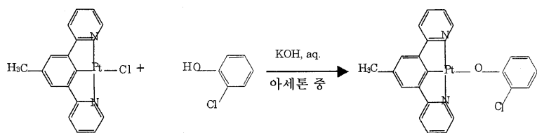
(합성예 33)
