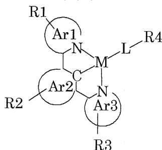
화학식 1
