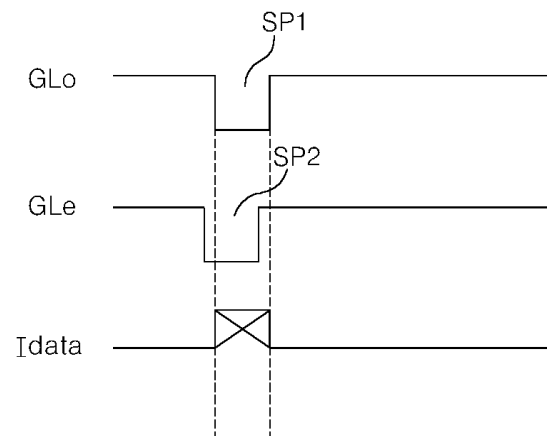
도면4
